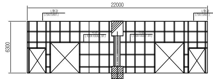
단면 B-B
