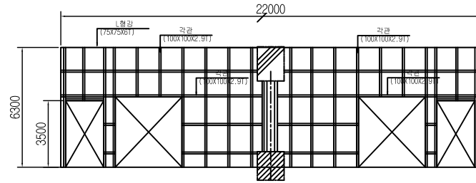
단면 B-B
