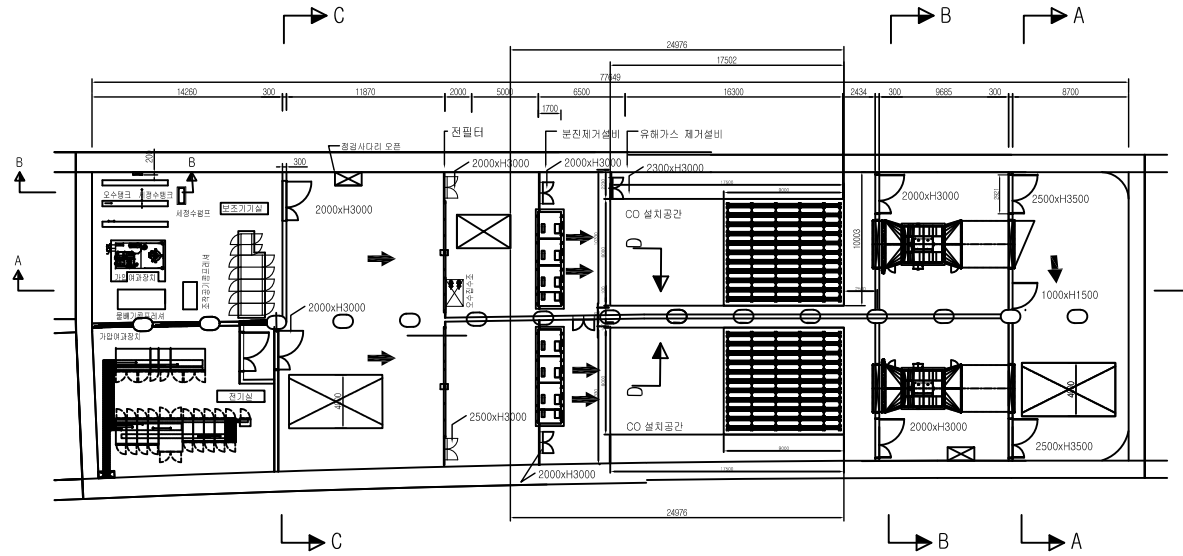
격벽 설치 상세
