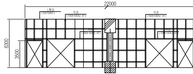
단면 A-A
